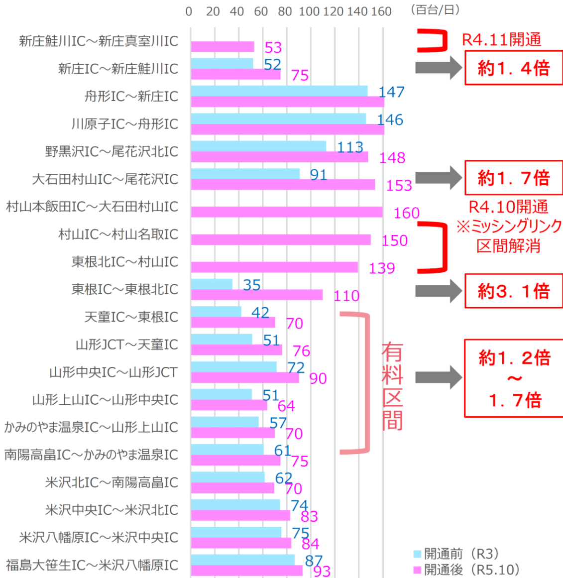
■東北中央自動車道の区間別交通量の変化（平日） ■断面交通量の変化（平日）
