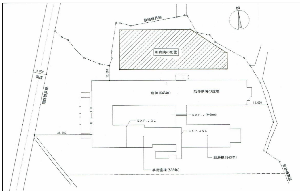
【 配置計画 】
