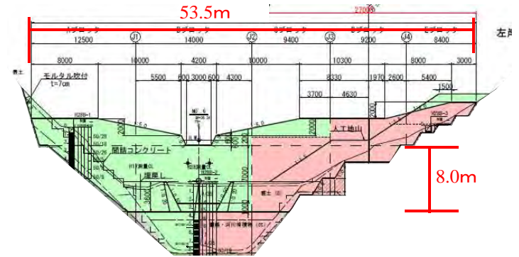
第2号えん堤正面図
