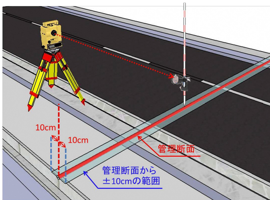
図 3-2 管理断面として入力したラインから道路延長方向に±10 cmの範囲
