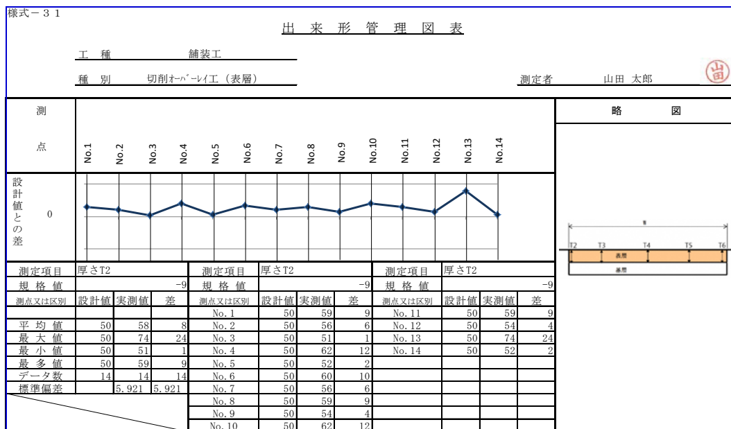
図6-1 出来形管理図表 作成例
