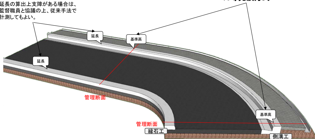
図 1-3 TS等光波方式とその他計測方法との組み合わせ例
