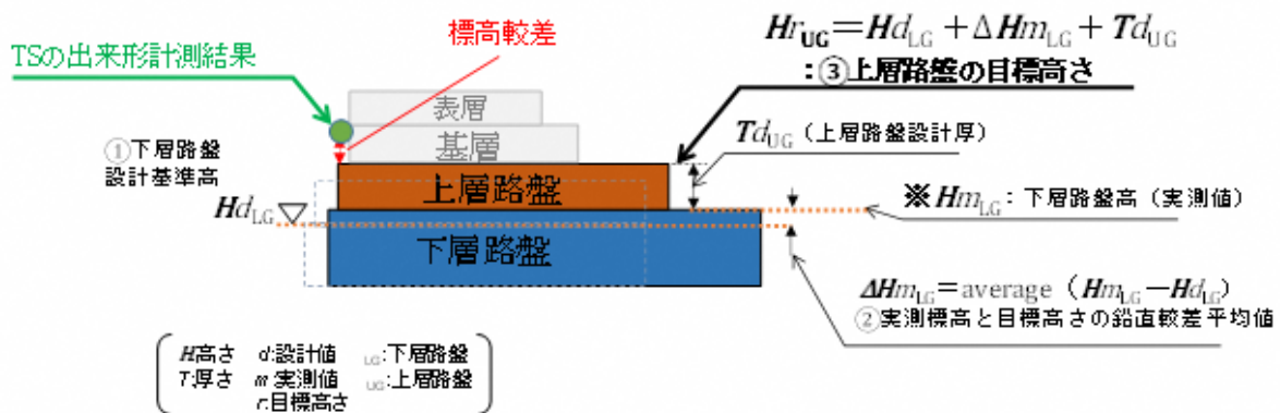
参考資料図4-1 上層路盤の目標高さ
