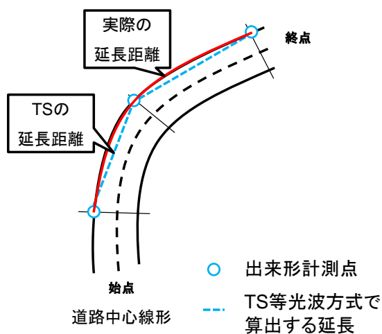
図 1-2 延長計測の留意事項
