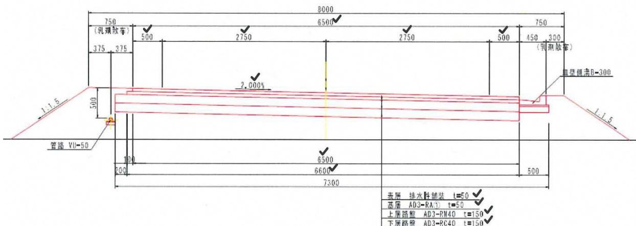
標準横断図 s=1:30
