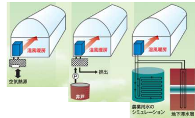
熱源：空気 熱源：地下水等 ヒートポンプシステム
