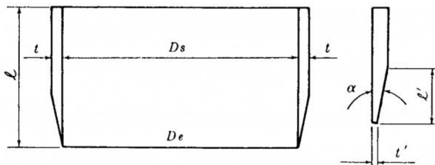
図 3 - 1 サンプリングチューブ
