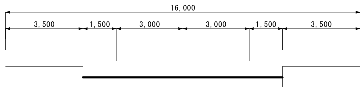
計画横断図
