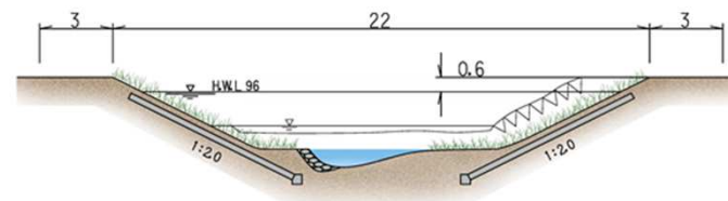
河川整備計画断面図
