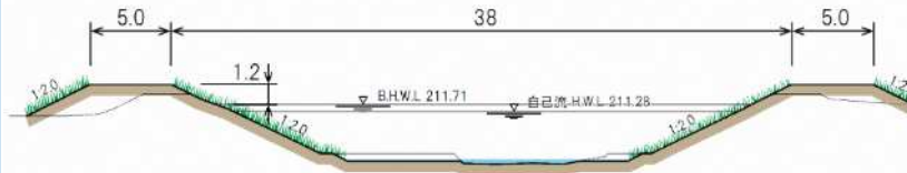
河川整備計画断面図 (最上川合流点から上流2.8km)
